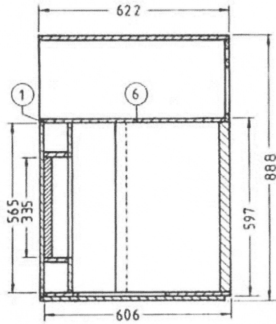
Schnitt A-B
